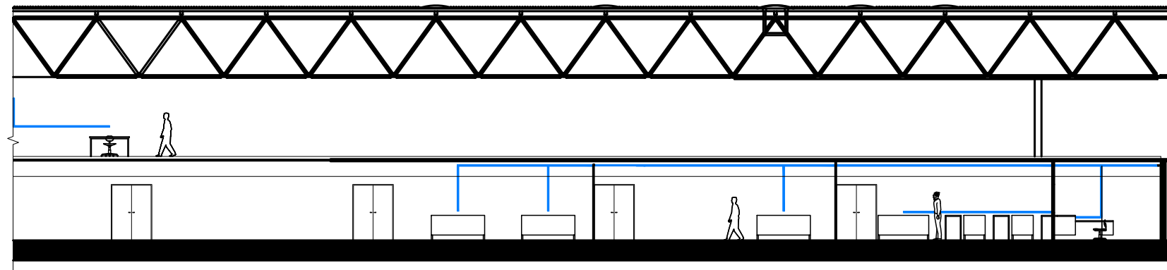
CORTE HH ESCALA 1:200
