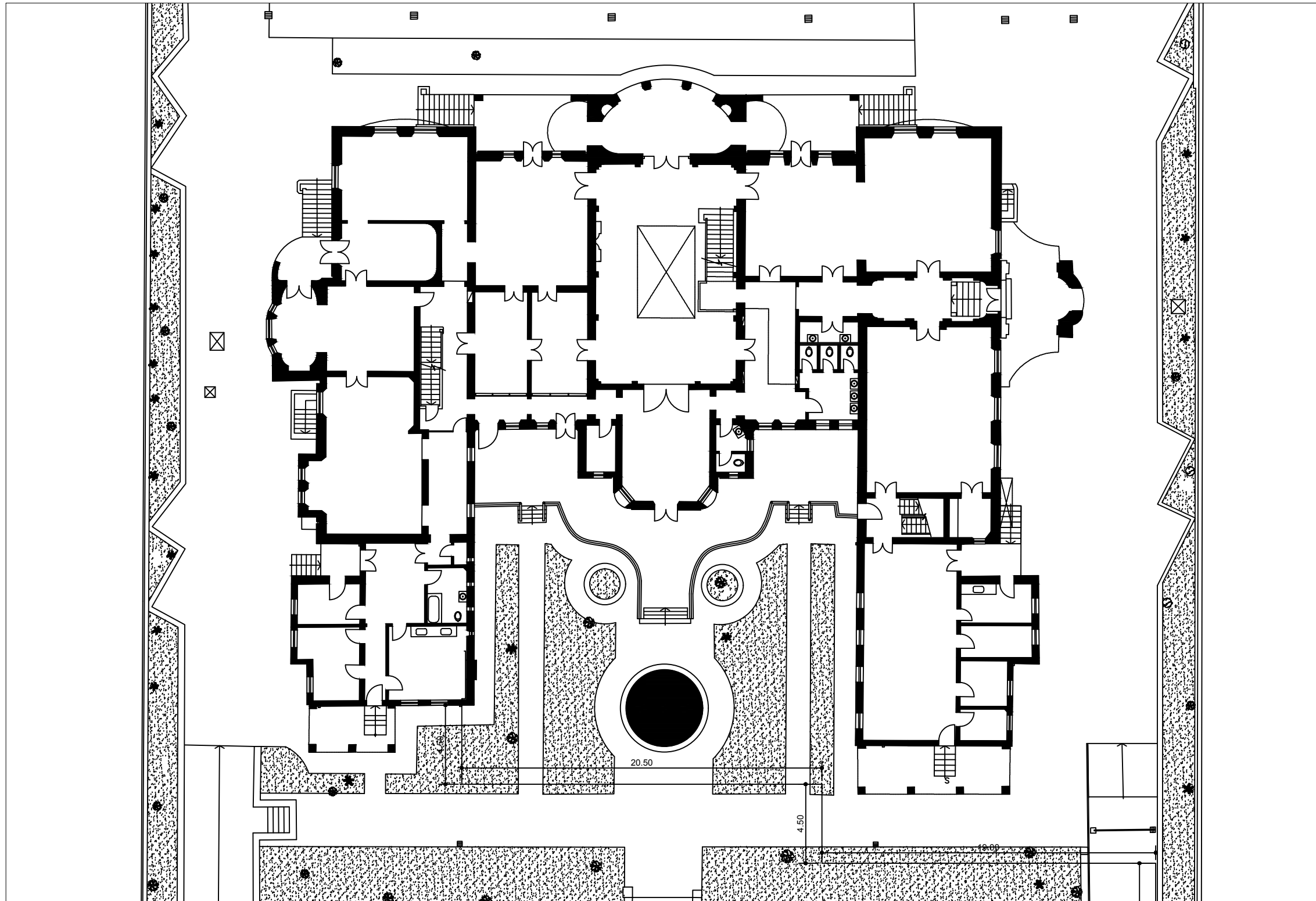
térreo 1:250
